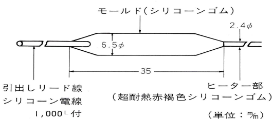
ベルトヒーター
