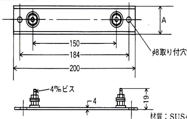
寸法図 (mm)
